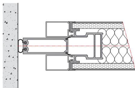
Montant Télescopique
