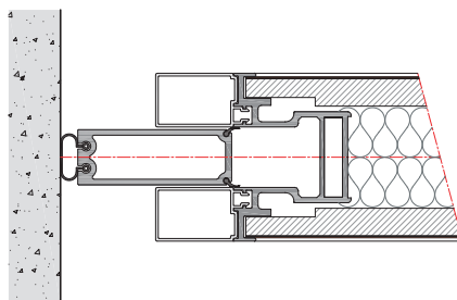
Montant Télescopique
