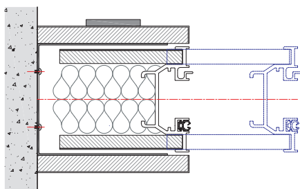
Profil d'Ajustement Télescopique Electrique
