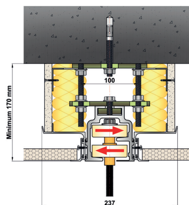
Rail en caisson
