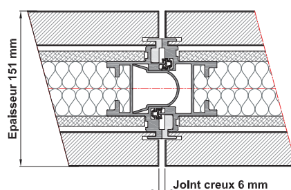
Jonction de Panneaux
