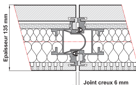
Jonction de Panneaux
