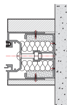
Profil d'Ajustement Latéral
