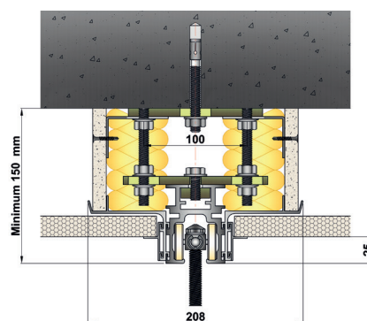
Rail encastré dans plafond suspendu (avec barrière phonique)
