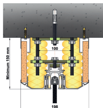
Rail en caisson
