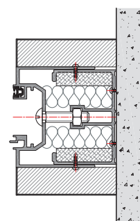
Profil d'Ajustement Latéral
