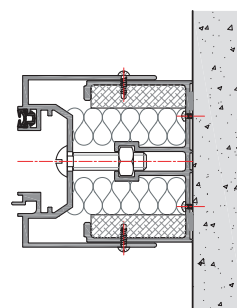
Profil d'Ajustement Latéral
