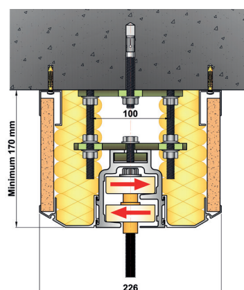
Rail en caisson
