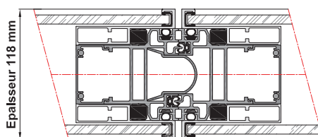
Jonction de Panneaux
